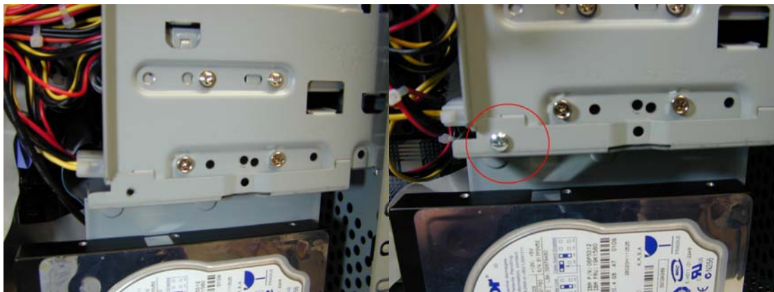
(圖 10，圖 11)「Second HDD Tray」上端也可緊密結合，請鎖上螺絲固定。
