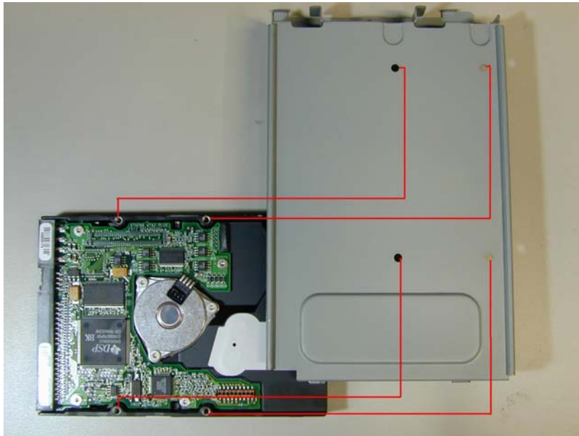
(圖 3) 將螺絲依指示鎖在背面
